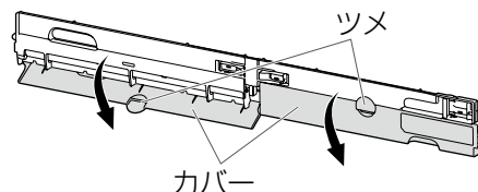
カバー
