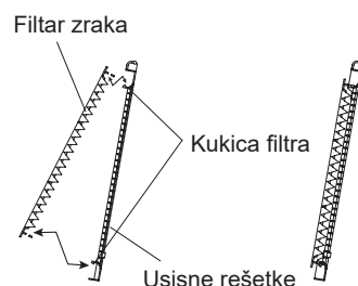
Usisne rešetke
